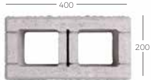
Pustak podmurówkowy - rozszczepiany z dwóch stron
